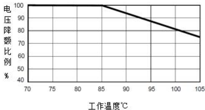
额定电压降额曲线
