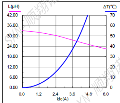
SMMS1040-101M
