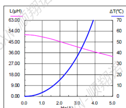
SMMS1040-470M
