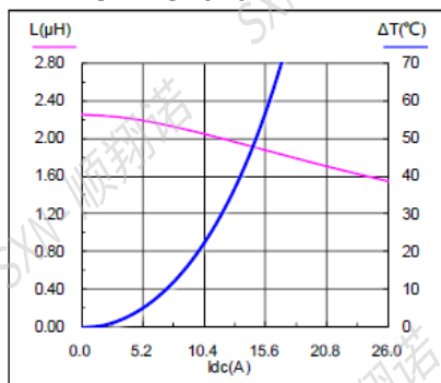
SMMS1040-2R2M
