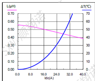
SMMS1040-R56M
